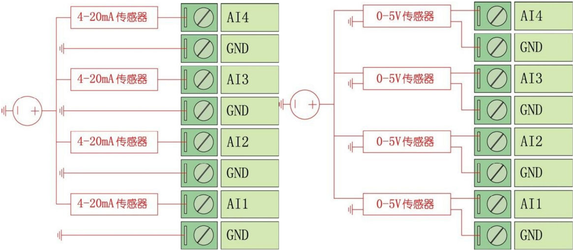
4~20mA 电流信号输入
